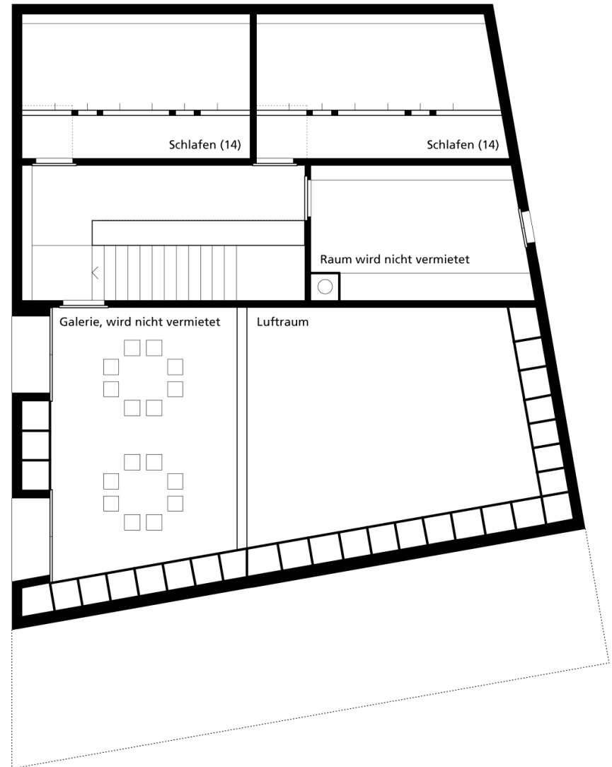
Obergeschoss Pfadiheim Baregg Baden
