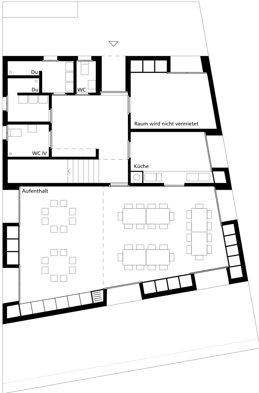
Erdgeschoss Pfadiheim Baregg Baden
